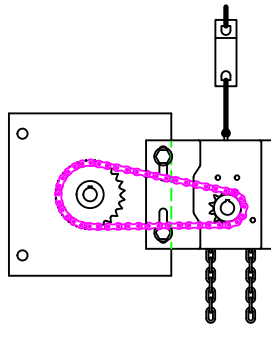
Type FHCM
